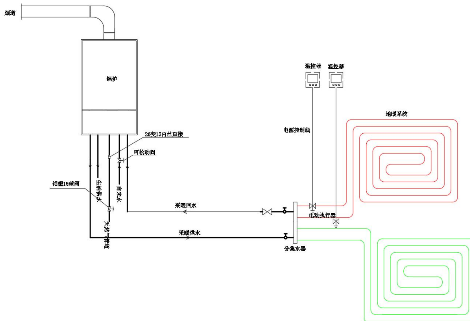
水暖采暖示意图
